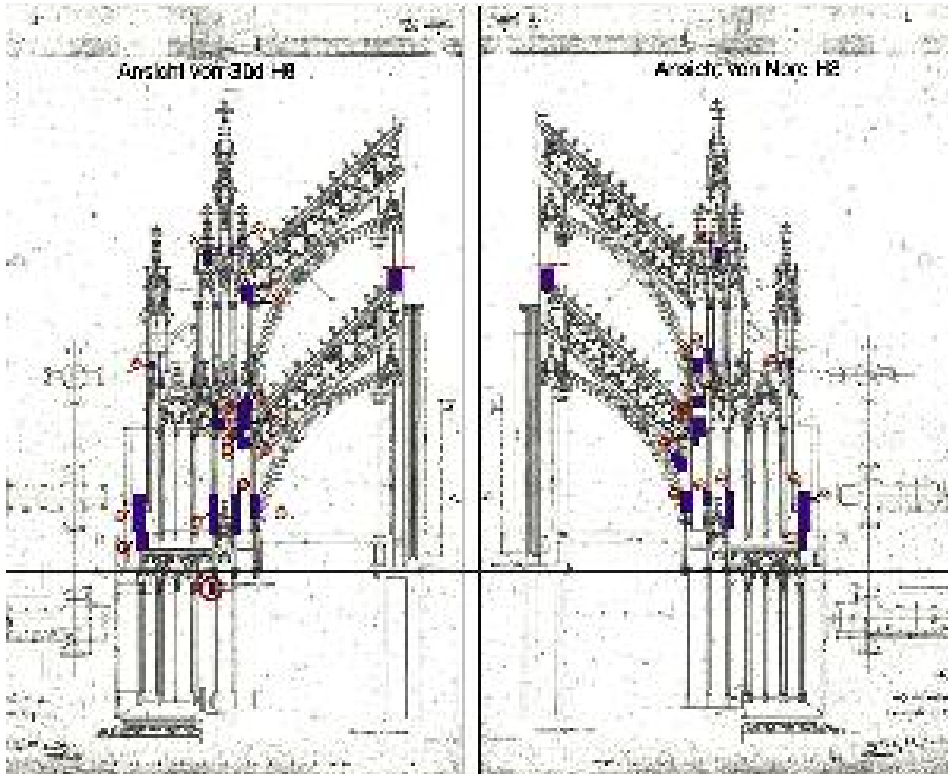
2. Matthias Hofmann, Dokumentation der ausstehenden Arbeiten am Strebewerk H 8–H 9.
