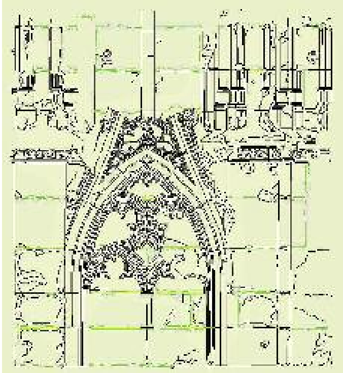
29. Norbert Nussbaum und Sabine Lepsky, Schadenskartierung am spätmittelalterlichen Pfeiler F 3.
